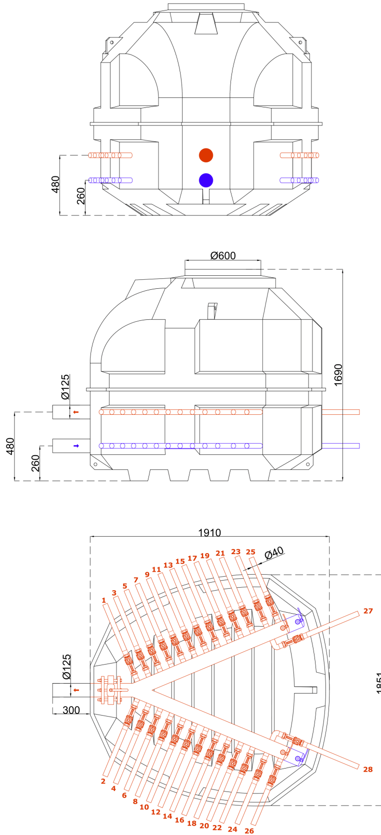
Rys. 17. Studnia Terra V-SERIES z rotametrami - 28 sekcji
