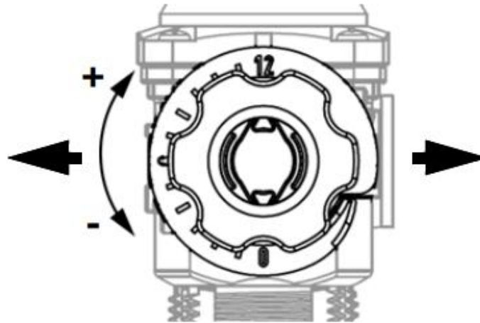
Rys. 25. Pokrętko rotametrów tworzywowych
