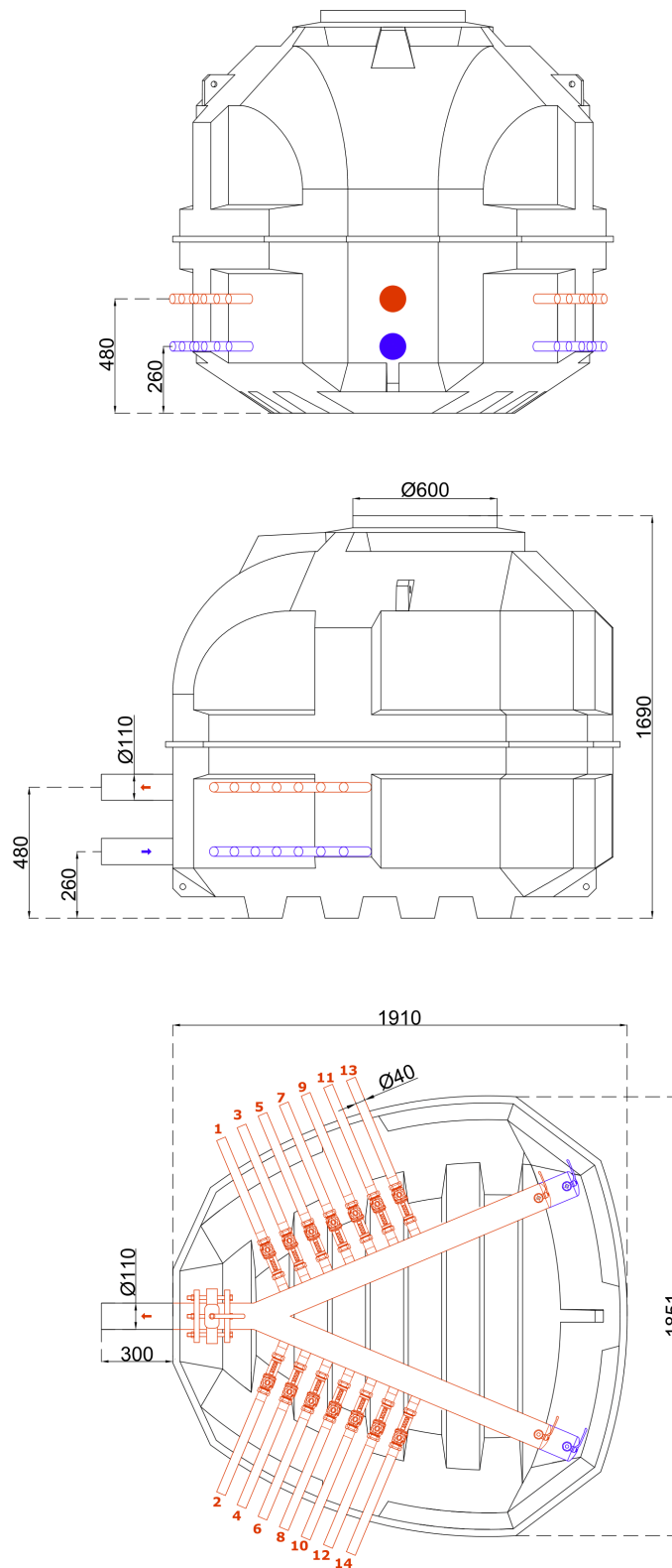
Rys. 3. Studnia Terra V-SERIES z rotametrami - 14 sekcji
