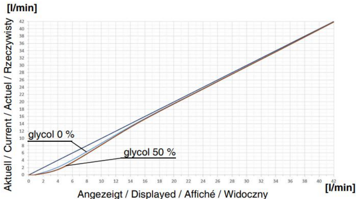
Rys. 27. Krzywe korekcyjne dla rotametrów tworzywowych
